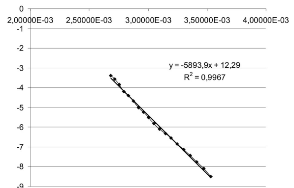
GAMBAR 2: Grafik \ln \sigma versus 1/T
