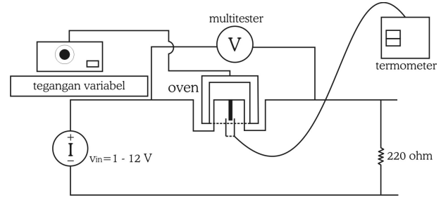
GAMBAR 1: Rangkaian pengukuran resistansi untuk berbagai suhu [5]
