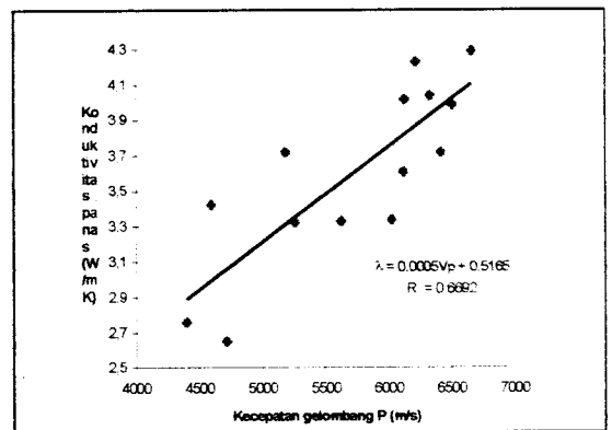
Gambar 3. Grafik relasi konduktivitas panas dengan kecepatan gel. P untuk sampel batuan vulkanik permukaan Tangkuban Perahu.
