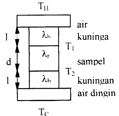
Gambar 1. Alat uji laboratorium untuk mengukur konduktivitas panas sampel batuan
