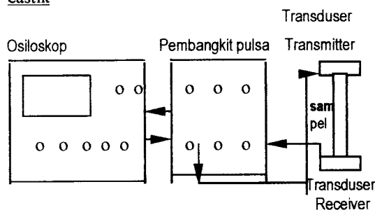
Gambar 2. Rangkaian alat pengukur kecepatan gelombang elastik
